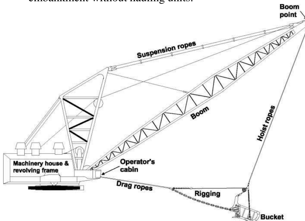
Fig. Dragline
